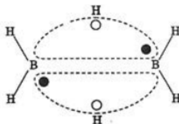
Fig. 5.4 Diborane
