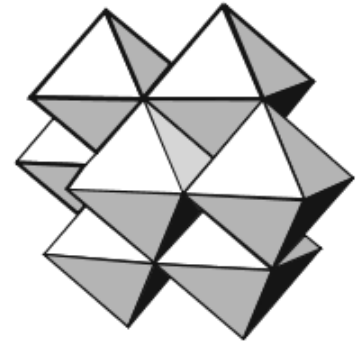
Fig. 5.30 (NH_4)_4 Mo_8O_{26} \cdot 5H_2O
