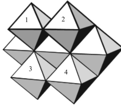
Fig. 5.29 [Mo_7O_{24}]^{6-}
