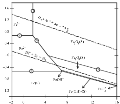
Fig. 3.20 Pourbaix pH Diagram of Fe
