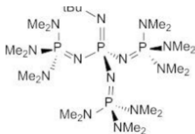
t-Bu-P4
