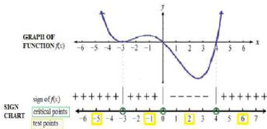
चित्र 4.1 बहुपद असमानता
